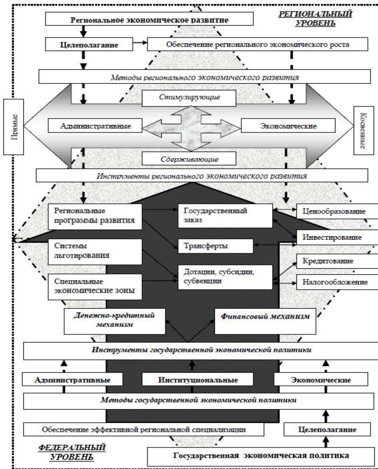
Рисунок 1 - Схема макроэкономического взаимодействия систем регионального экономического развития (разработано автором)
