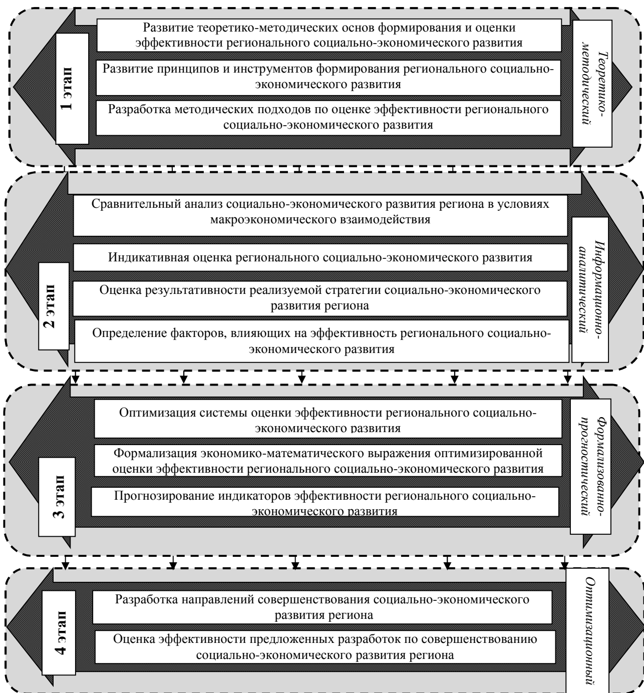
Рисунок 2 – Структурная схема рекомендуемой методики индикативной оценки планируемых разработок по совершенствованию социально-экономического развития региона (разработано автором)
